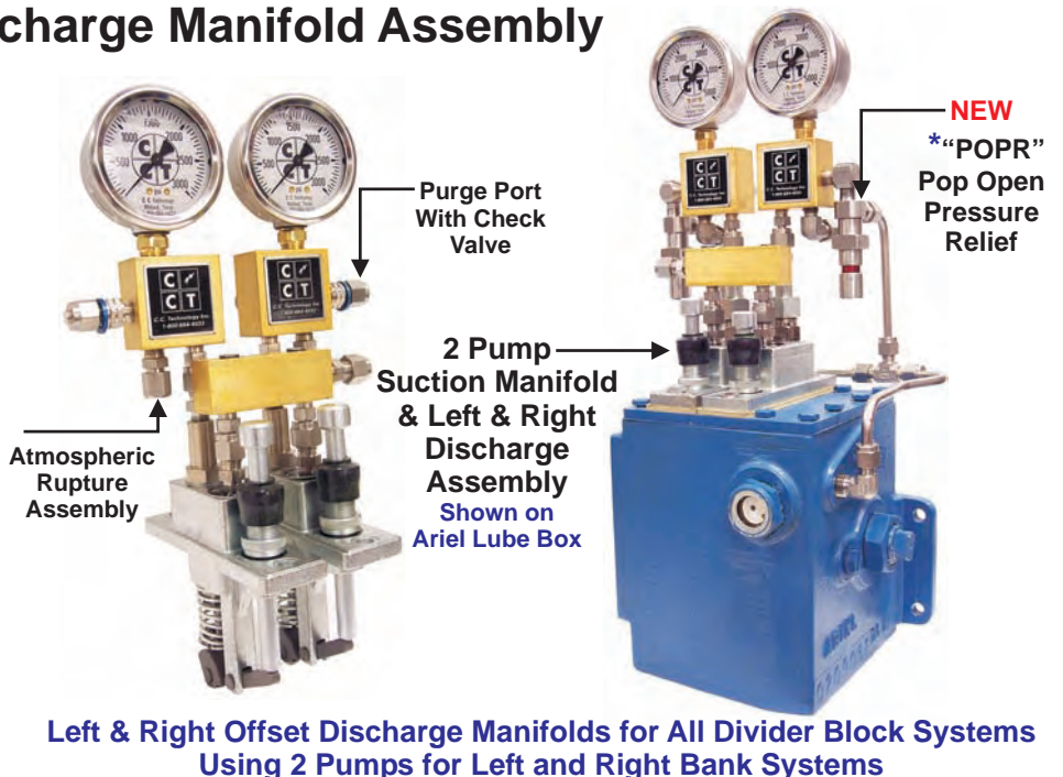
Part# 391040-L Left Part# 391040-R Right
